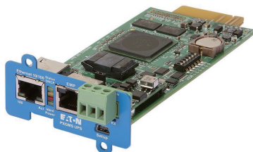
图5-5: PXGMS网卡
