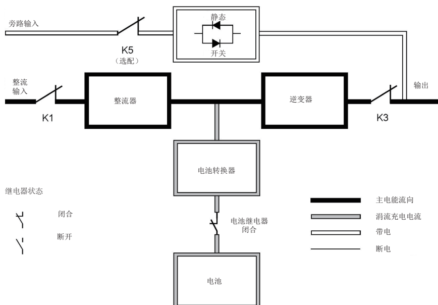
图2-5： 双转换模式下的电能通过UPS的路径
