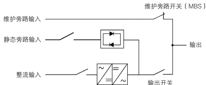
图6-52: 维护旁路模式下开关状态
