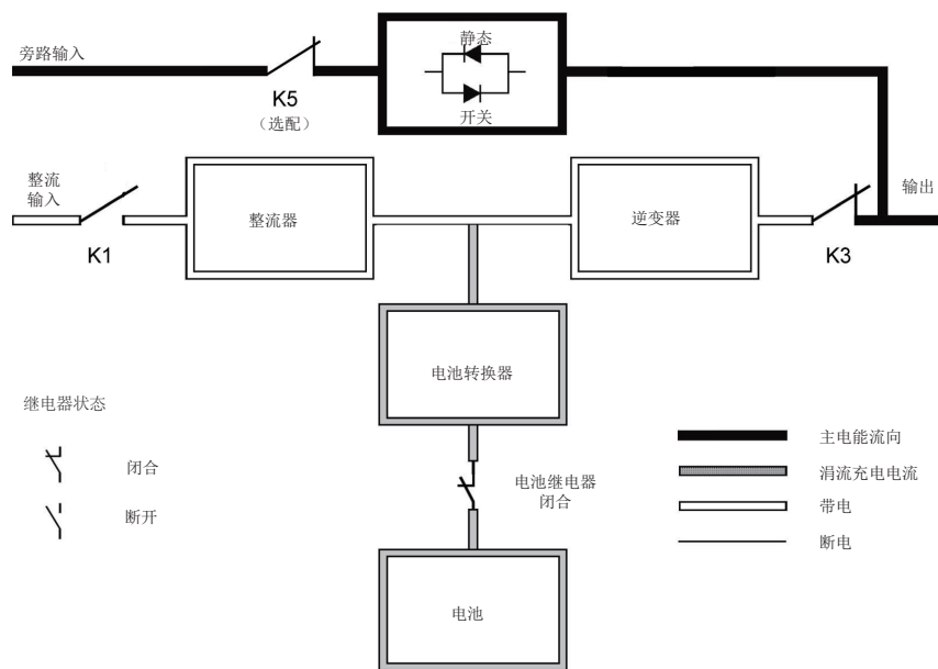
图2-6: ESS 模式下电能通过 UPS 的路径
