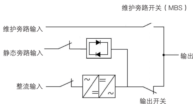
图6-53: 在线模式下开关状态
