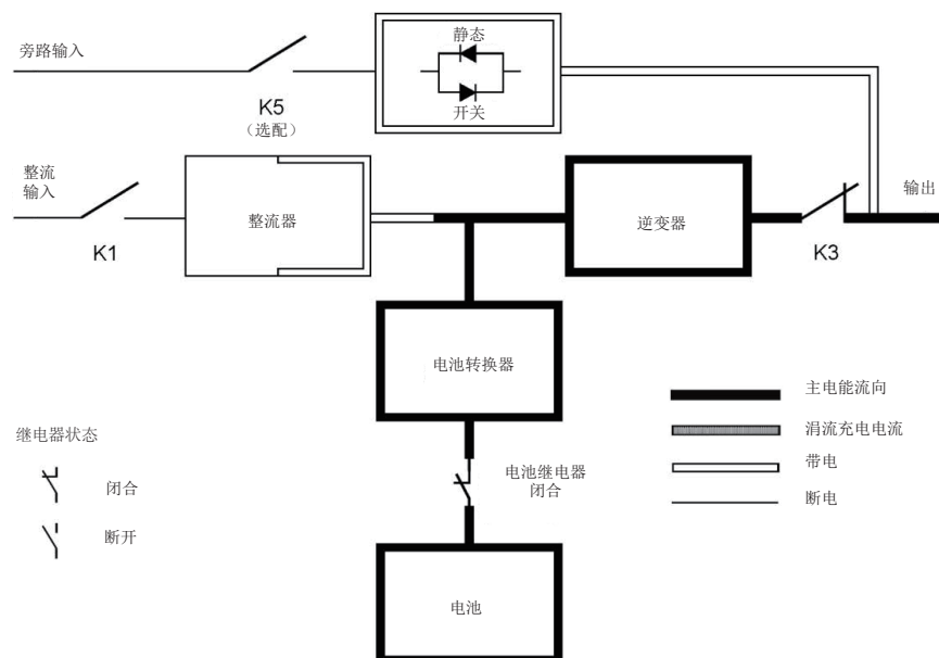
图2-7: 电池模式下电能通过 UPS 的路径
