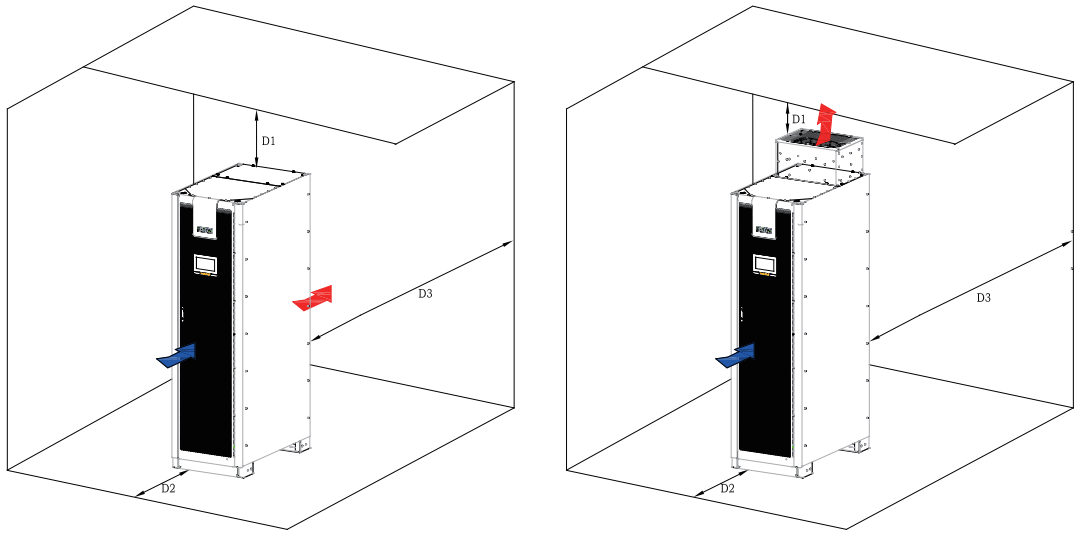
图3-1：UPS 机柜预留空间
