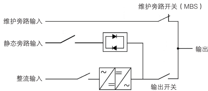
图6-51：维护旁路模式下开关状态
