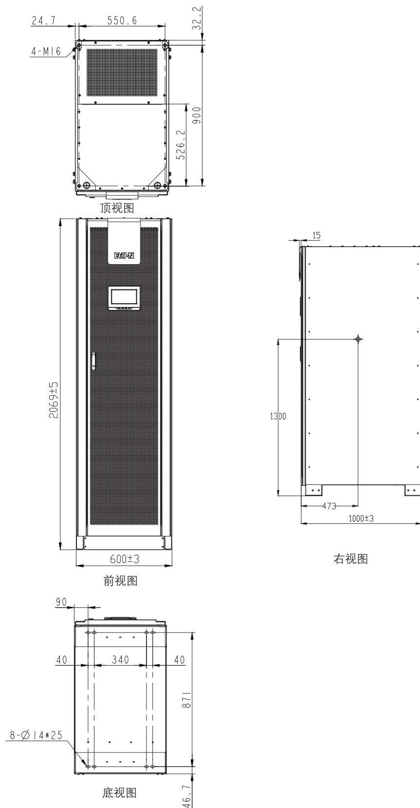
图3-2: UPS 尺寸重心图 (后出风)
