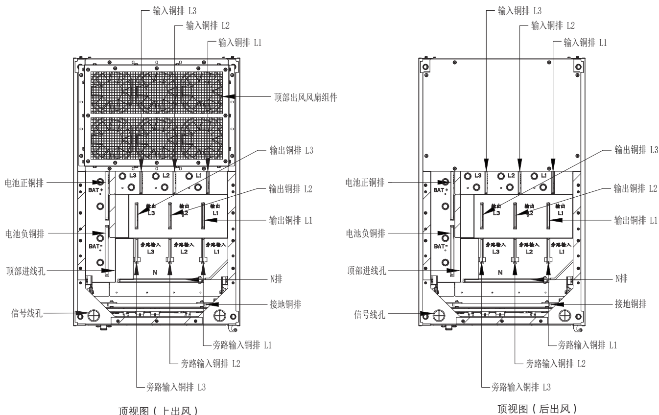
图4-10: 盖板 and 连接端子位置
