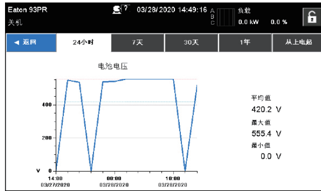
图6-23: 电压测量值屏幕
