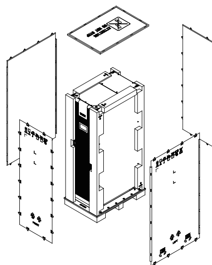
图4-2: 移除木箱
