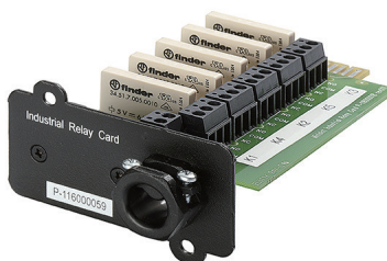
图5-7: 标准工业继电器卡
