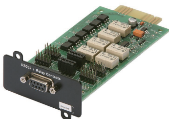
图5-6: 标准AS400/RS232卡
