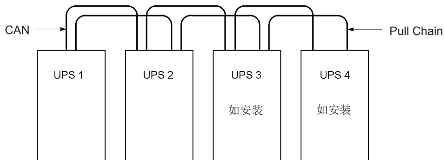
图4-16: 并机UPS系统的CAN和Pull-Chain的简化配线
