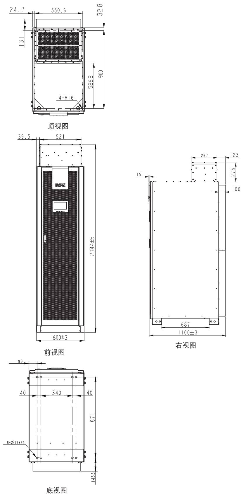
图3-3: UPS 尺寸图 (上出风)
