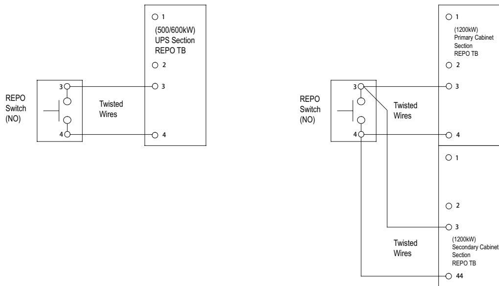
图4-13：常开 REPO 开关配线
