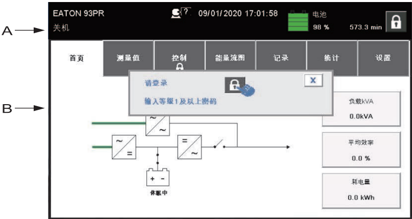
图6-3：触摸屏组成部分
