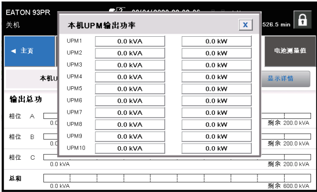
图6-20： 选择电压显示模式屏幕
