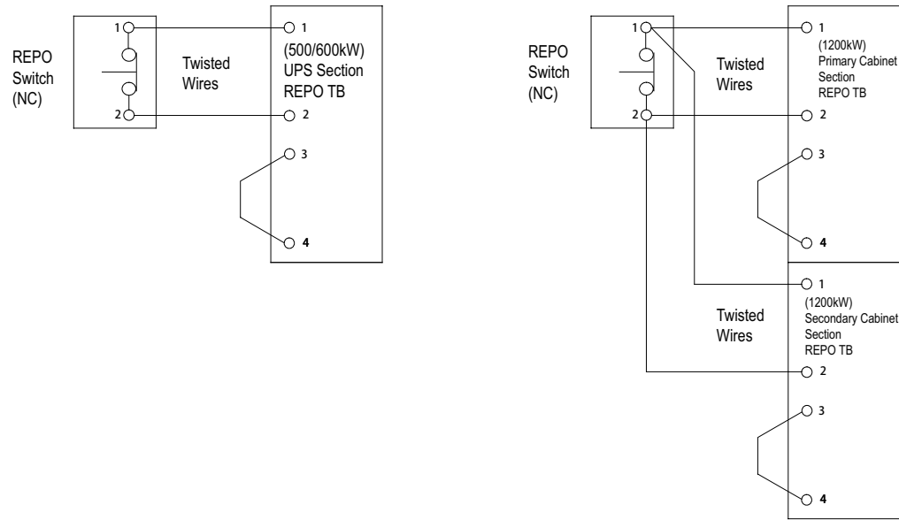
图4-14：常闭REPO 开关配线
