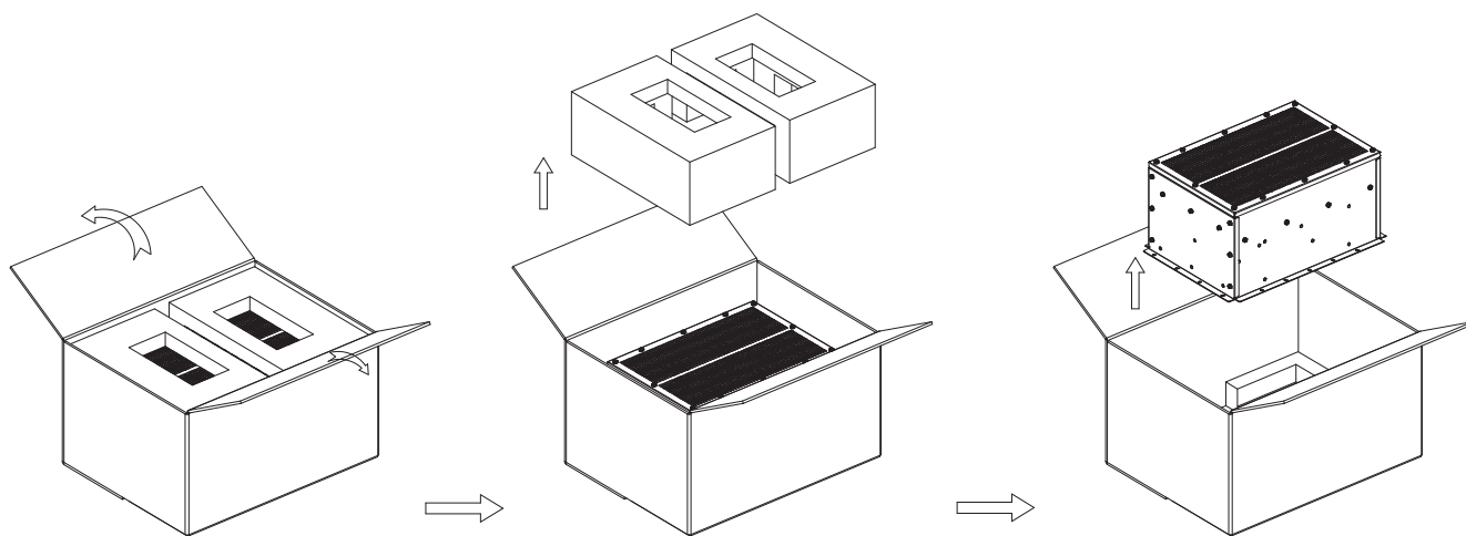
图4-7： 上出风组件包装拆卸
