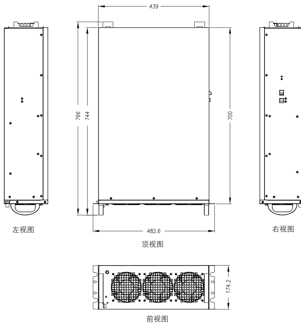
图3-4: UPM 尺寸
