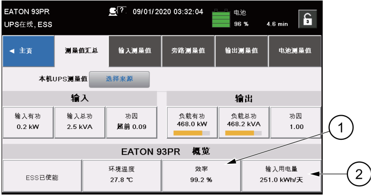
图6-9: 测量值汇总屏幕
