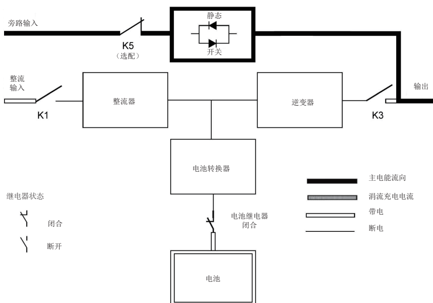
图2-8：旁路模式电能通过 UPS 的路径
