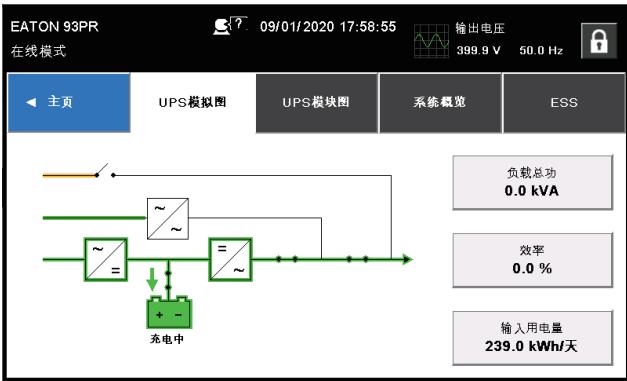
图6-37：UPS模拟图屏幕
