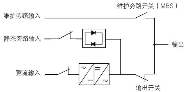
图6-50：在线模式下开关状态
