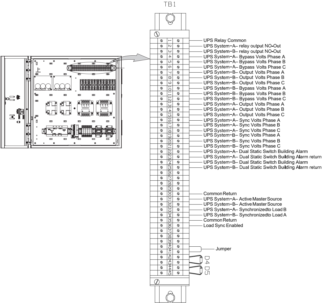
图4-18: 同步盒 TB1 端子位置
